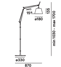
Tolomeo Basculante Floor
